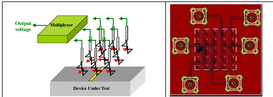
Figure 3 – Principe de la matrice de champ proche et motif de caractérisation en technologie HDI
